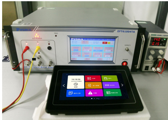
图 7-4 群脉冲测试图
